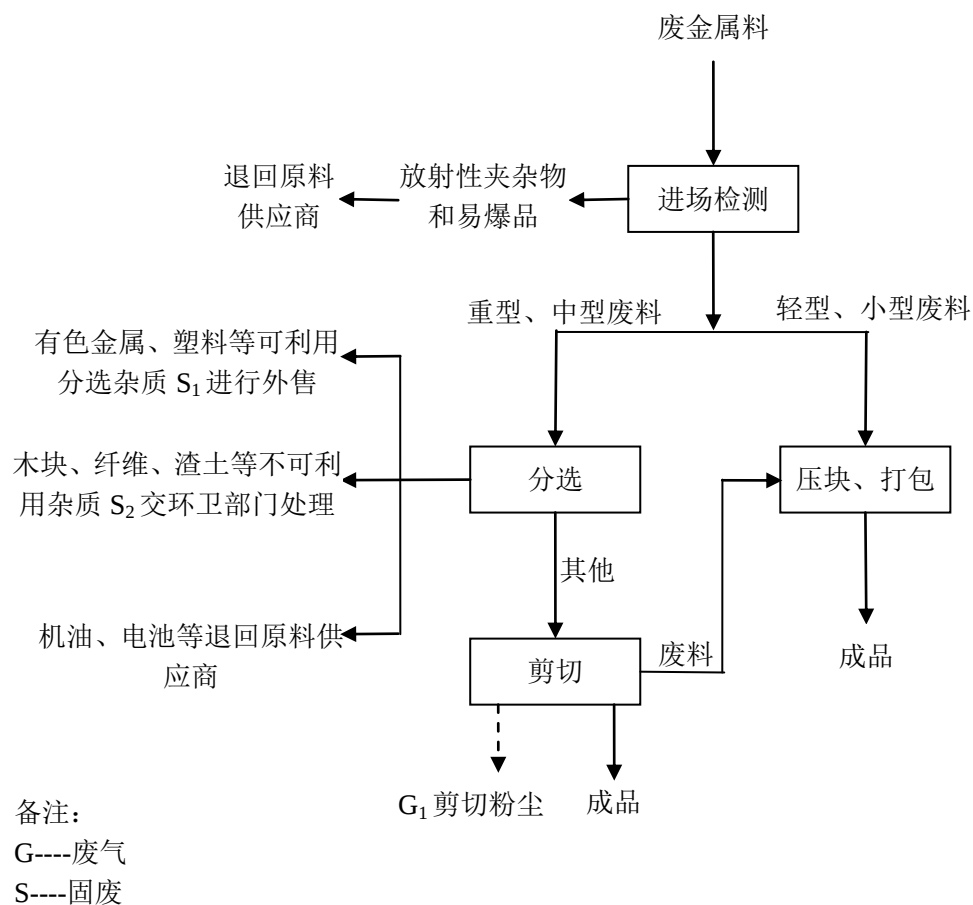
图 5-1 废不锈钢加工生产工艺流程及产污环节图
